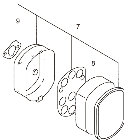
エアクリーナ詳細
