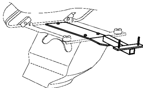
RXC, D, E型用本体取付金具（オプション）
