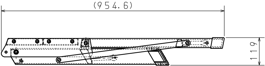
収納状態図
