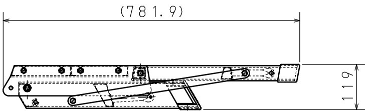
収納状態図
