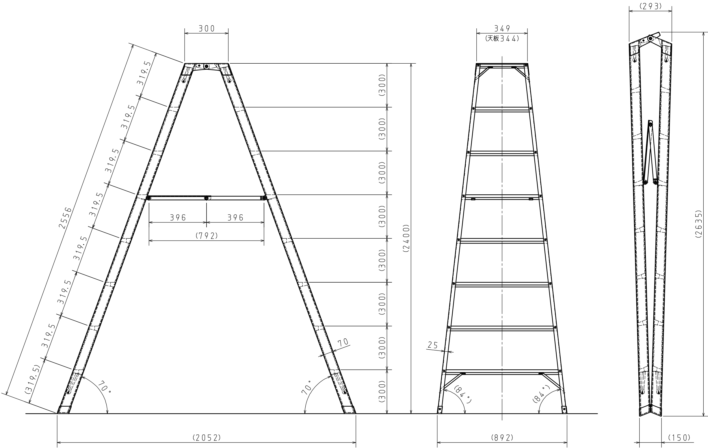
収納状態図
