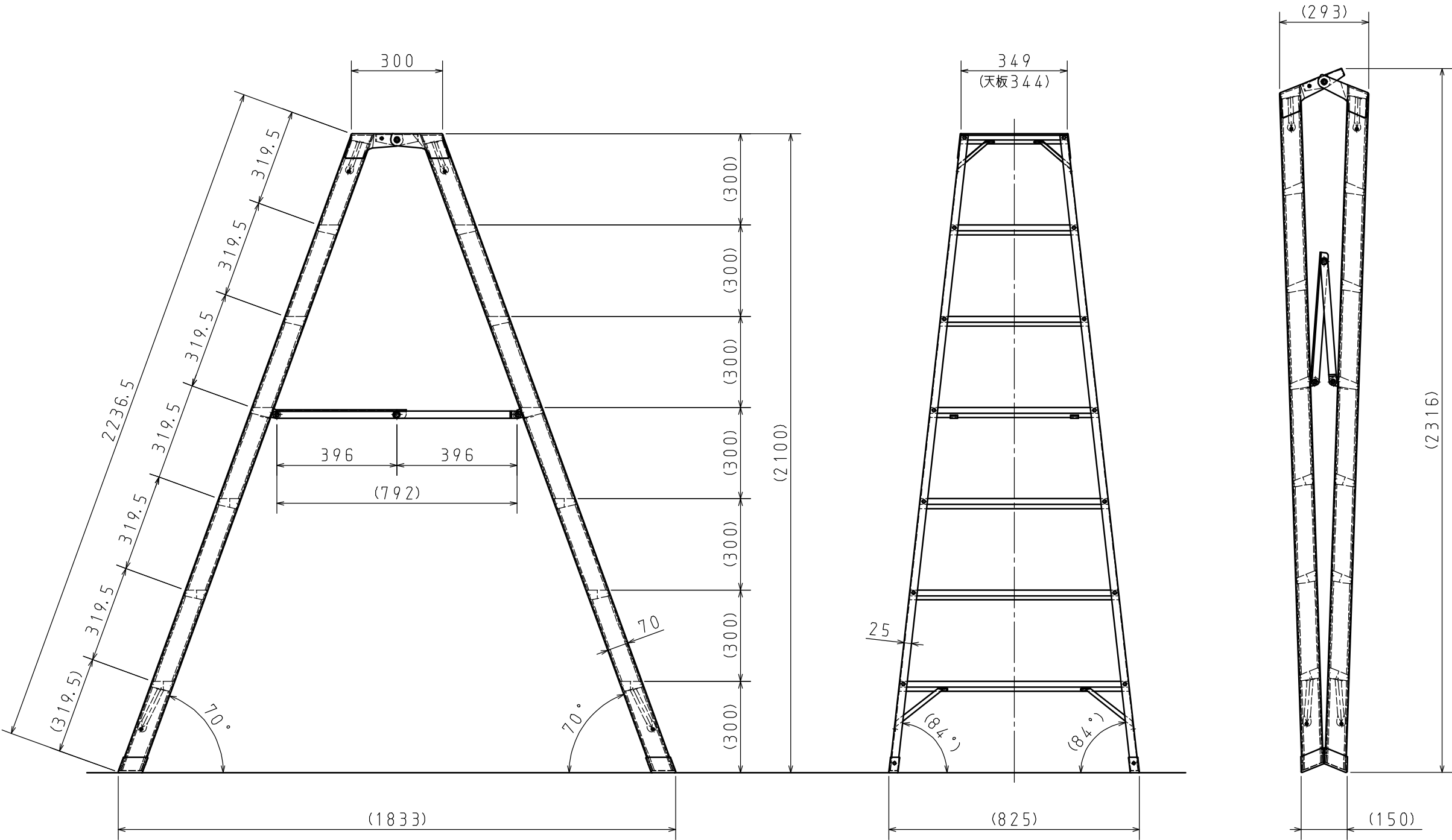
収納状態図
