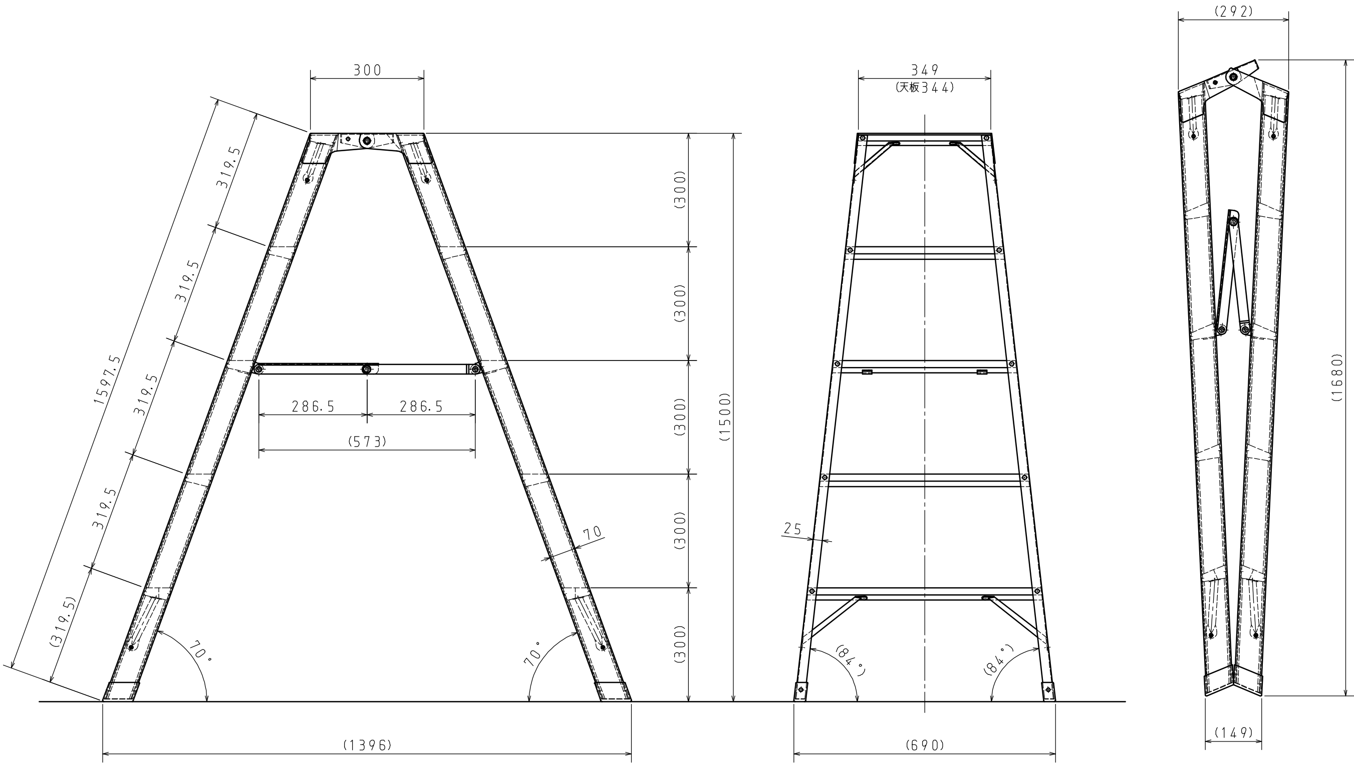
収納状態図
