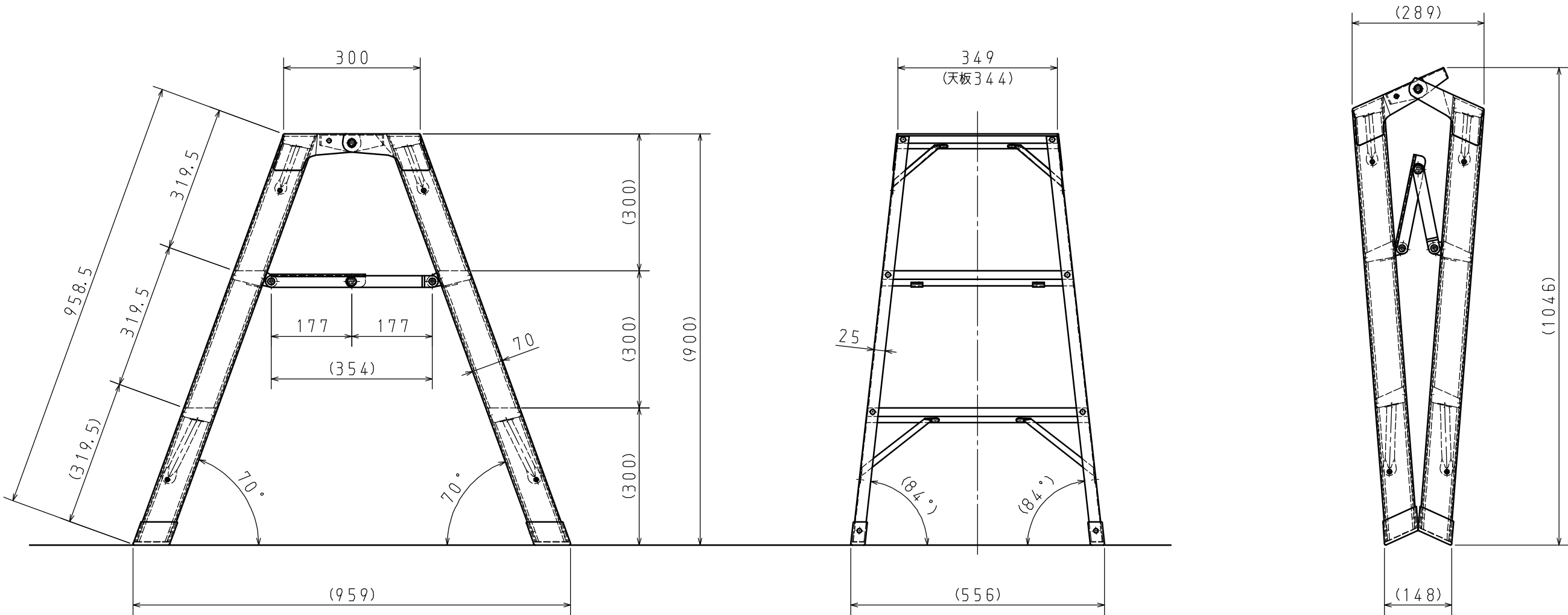
収納状態図
