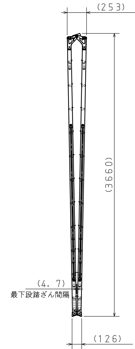
収納状態図 (S = 1 : 30)
