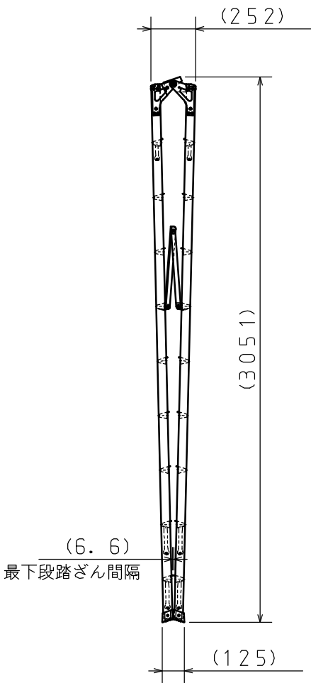
収納状態図 (S = 1 : 30)
