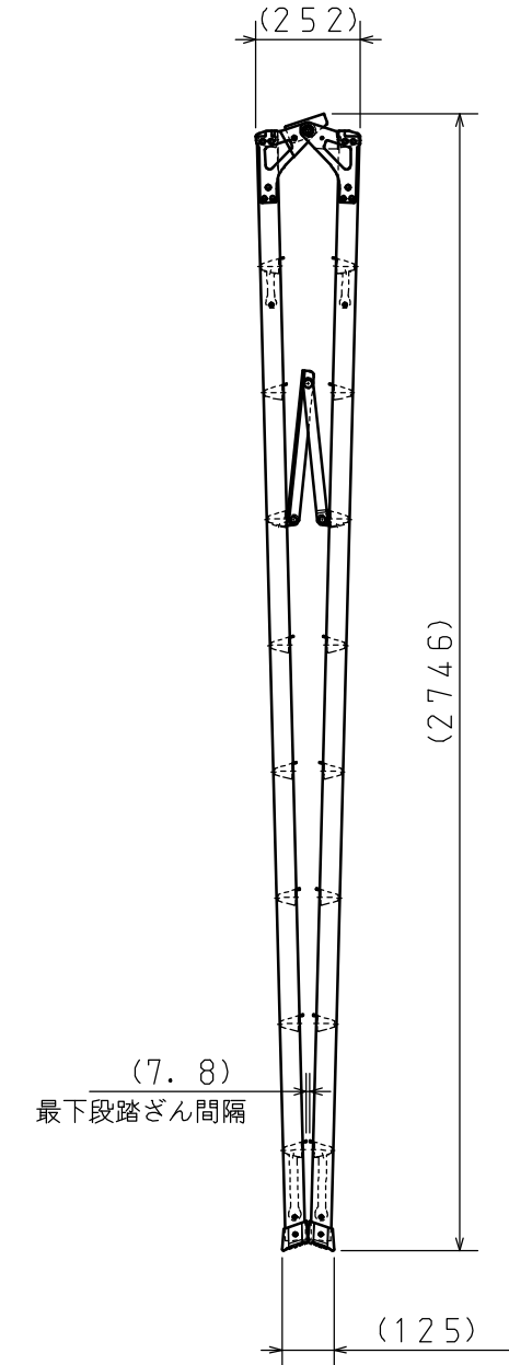
収納状態図 (S = 1 : 20)
