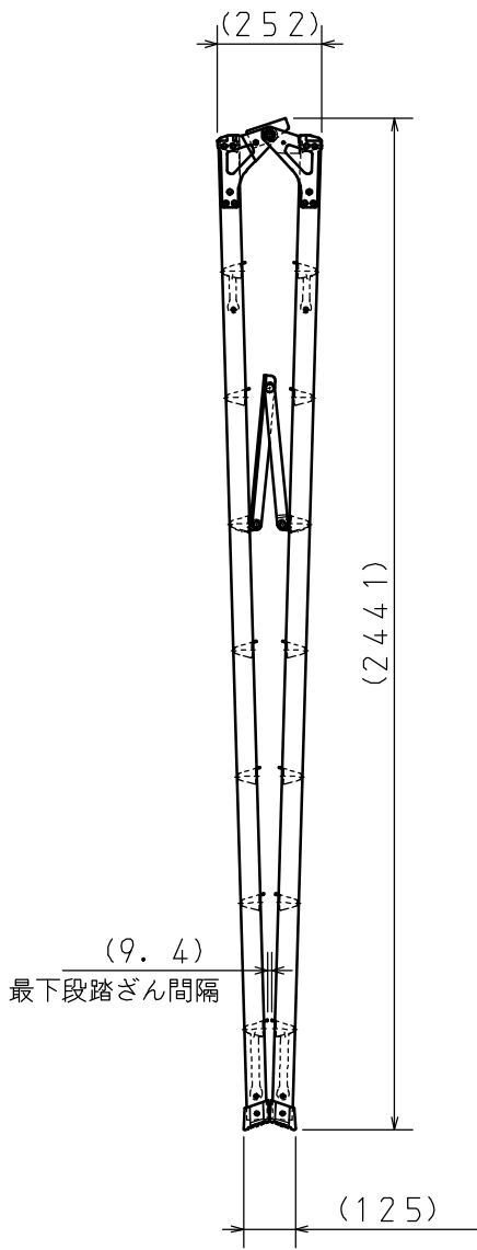
収納状態図 (S = 1 : 20)
