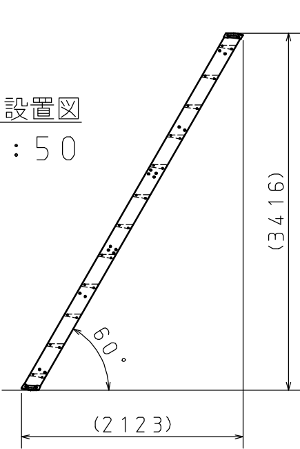
70°設置図 S = 1 : 50
