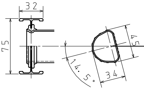
支柱・踏ざん詳細
