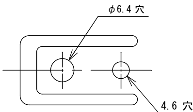
d部詳細図 (S=1:1)
