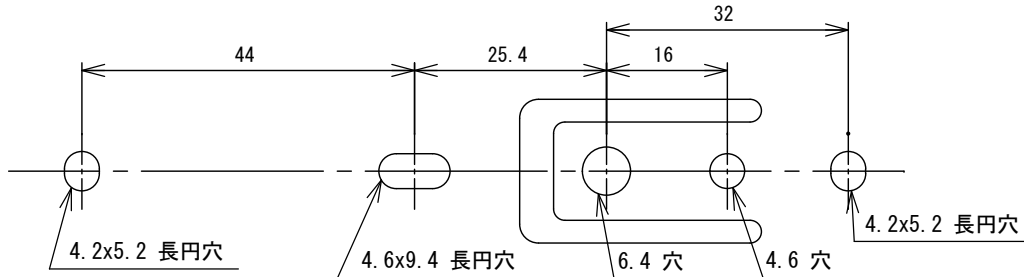
c部詳細図 (S=1:1)
