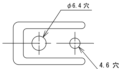
d部詳細図 (S=1:1)
