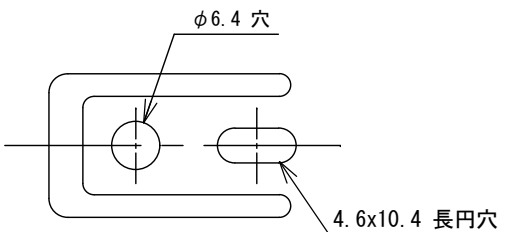
b部詳細図 (S=1:1)
