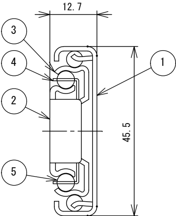
側面図 (S=1:1)
