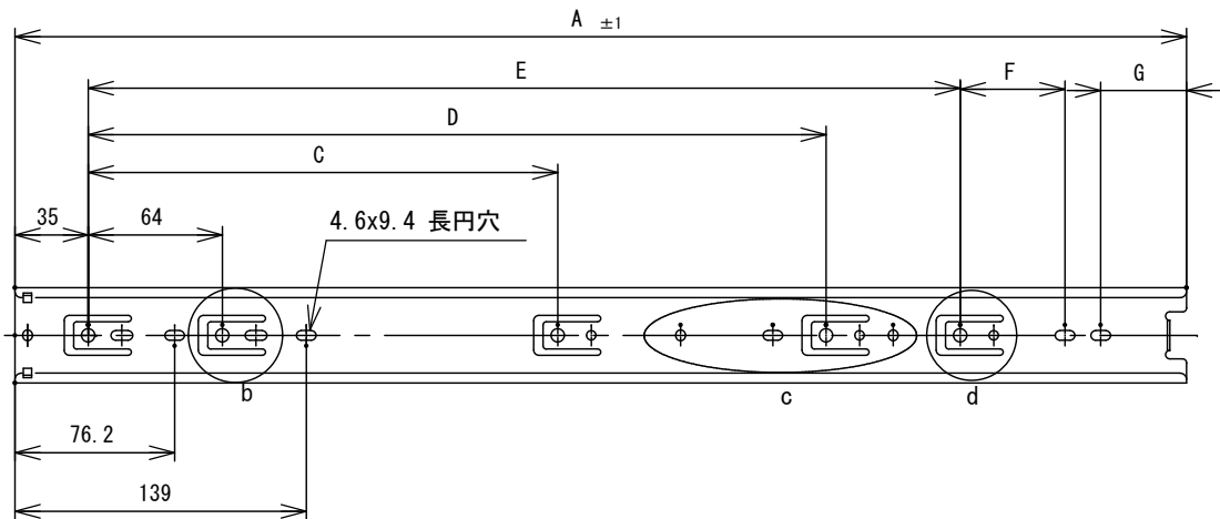
アウターメンバー穴位置
