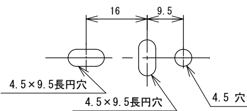
a部詳細図 (S=1:1)
