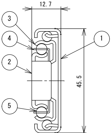
側面図 (S=1:1)
