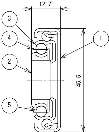
側面図 (S=1:1)
