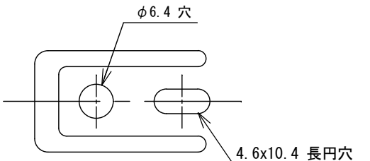
b部詳細図 (S=1:1)
