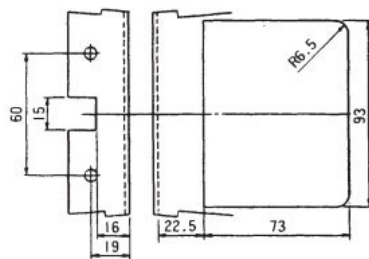
取付穴図
