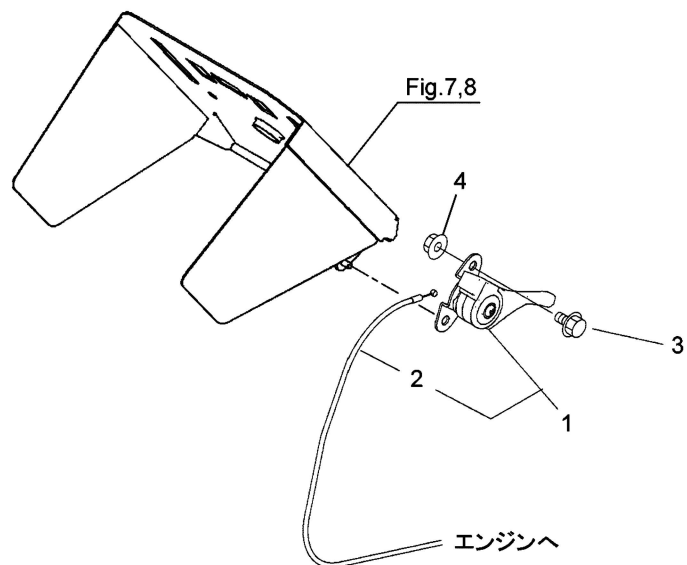
A詳細
