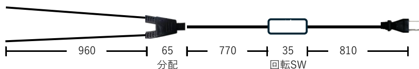
LED電気ローソク2灯（全長約2640mm）
