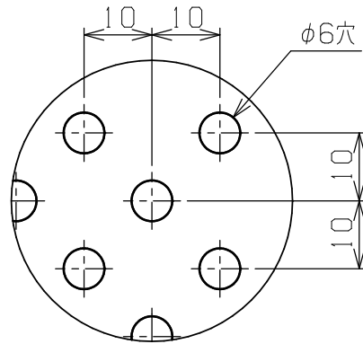
パンチング詳細 (S=1:1)
