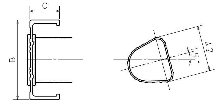
支柱及び踏ざん断面図 (S = 1 : 2)
