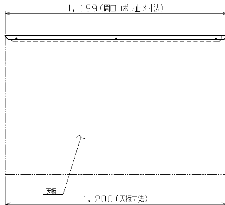
取付例 (S=1/12)
