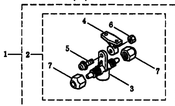
KIT(69) 細霧ノズル
