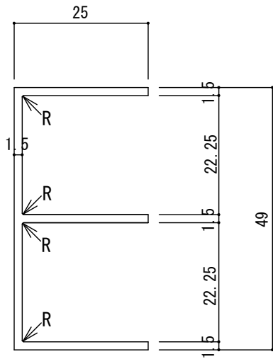
T0-174UP（上部レール用）色グレー
