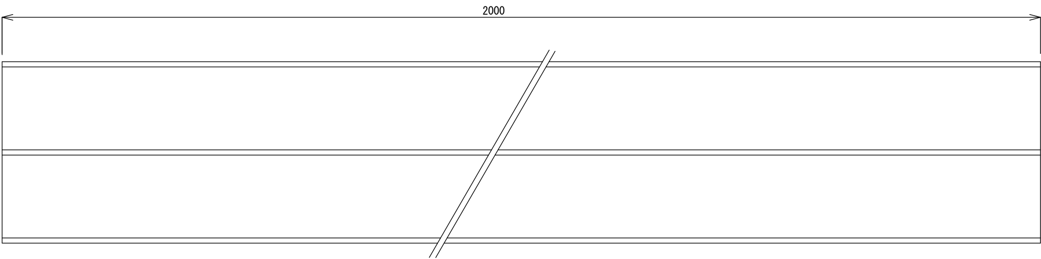
T0-174LP（下部レール用）色グレー
