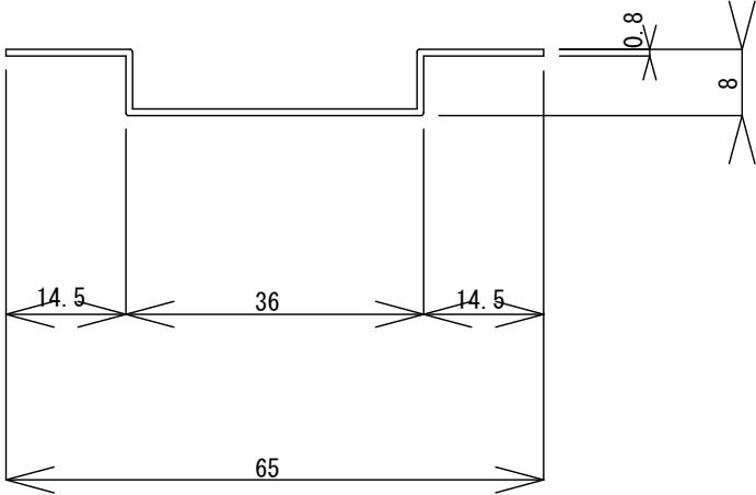
T0-84S、T0-84L共通断面図
