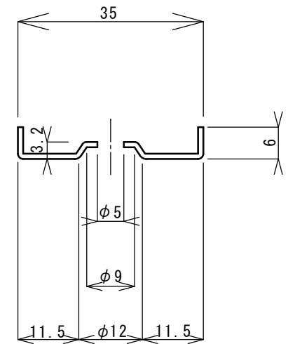
ヒース穴断面図
