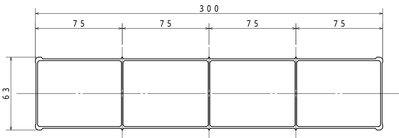
STXD型 断面図 (S=1:2)
