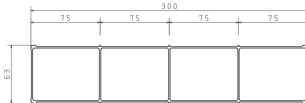
STXD型 断面図 (S=1:2)
