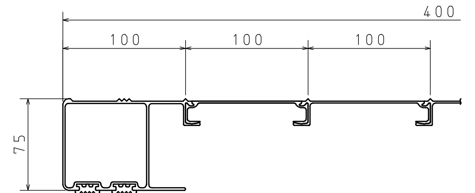
形材断面図 (S = 1 : 3)
