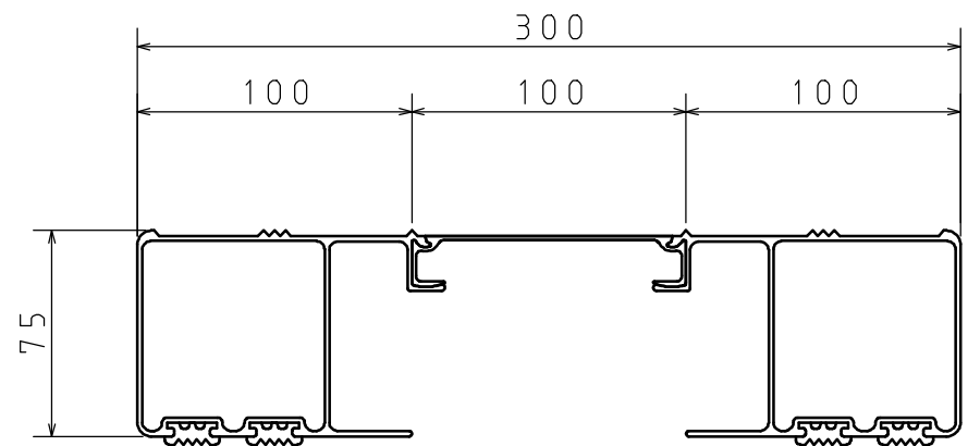
型材断面図 (S = 1 : 3)
