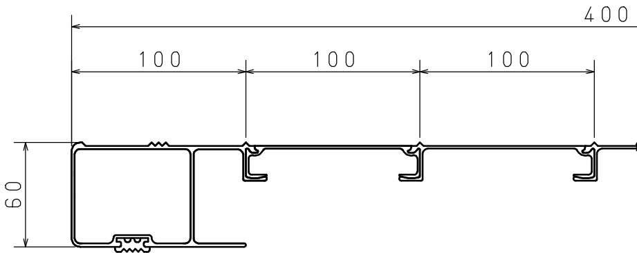
型材断面図 (S = 1 : 3)
