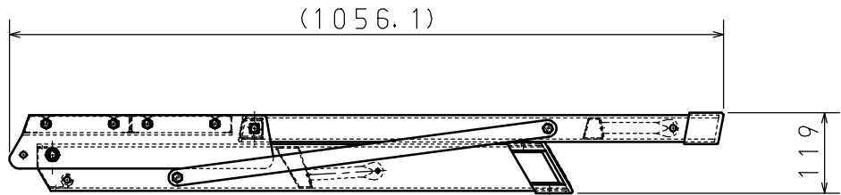
収納状態図
