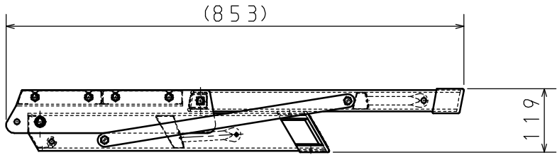
収納状態図
