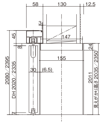
縦断面図
