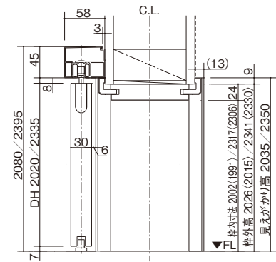
縦断面図
