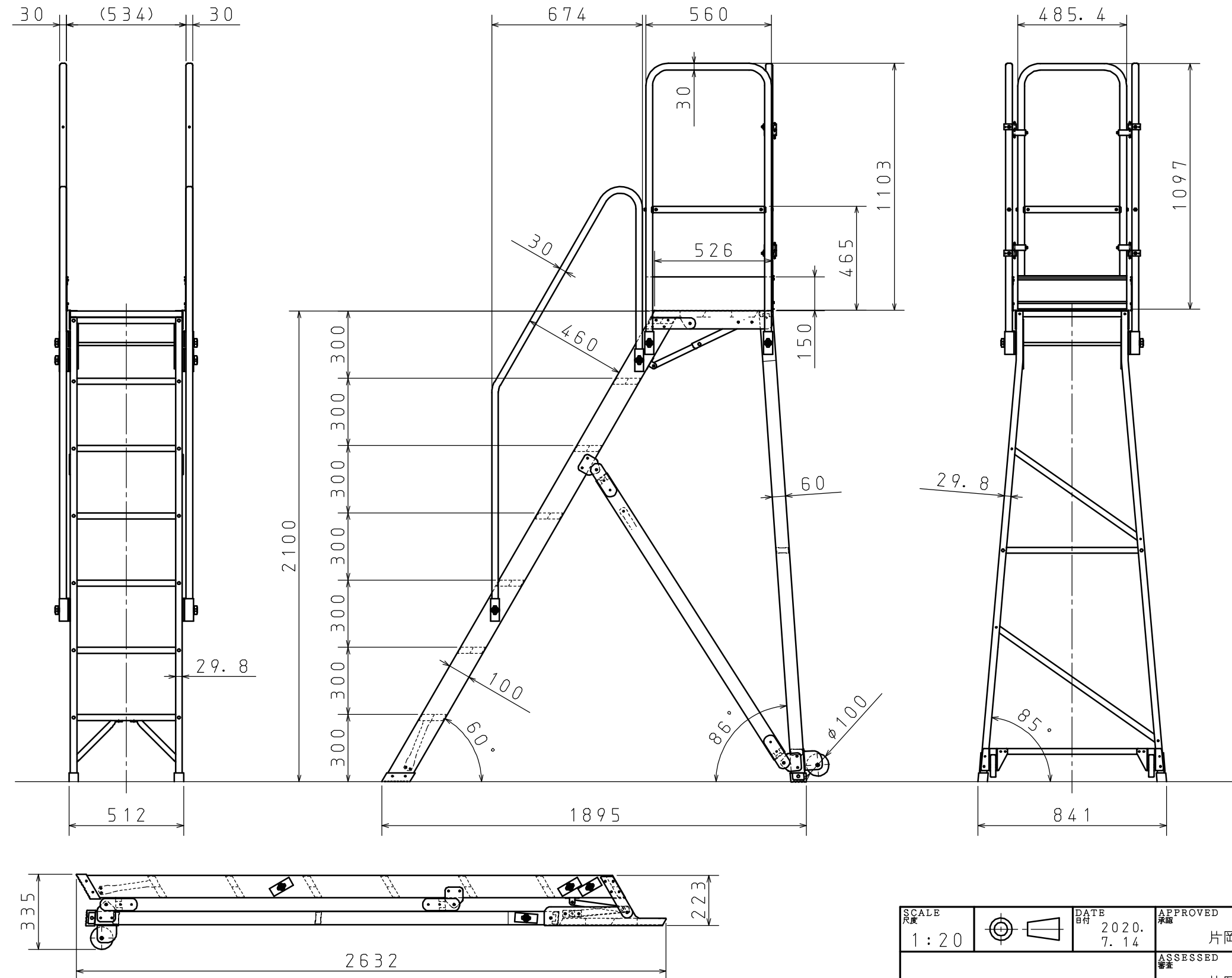
収納状態図
