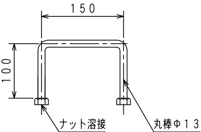
取手寸法（落込取手・浮上取手）
