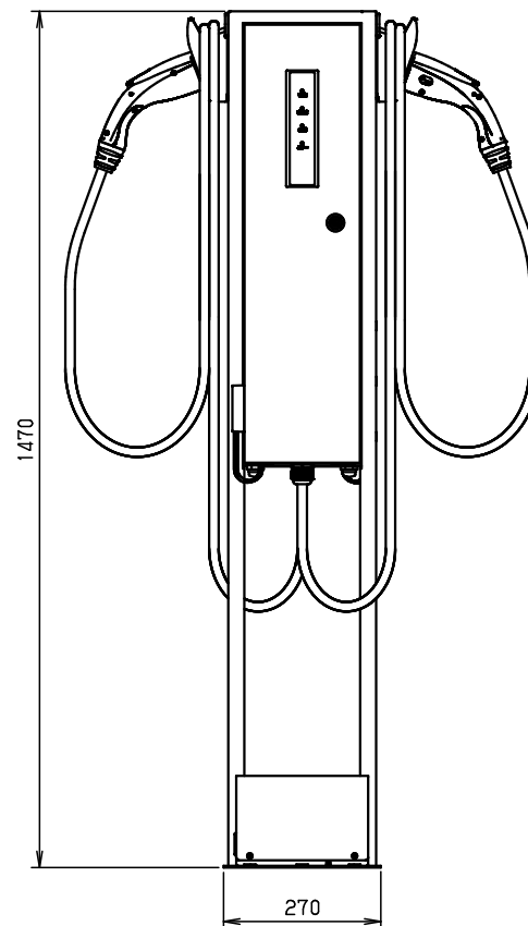
2台取付例
