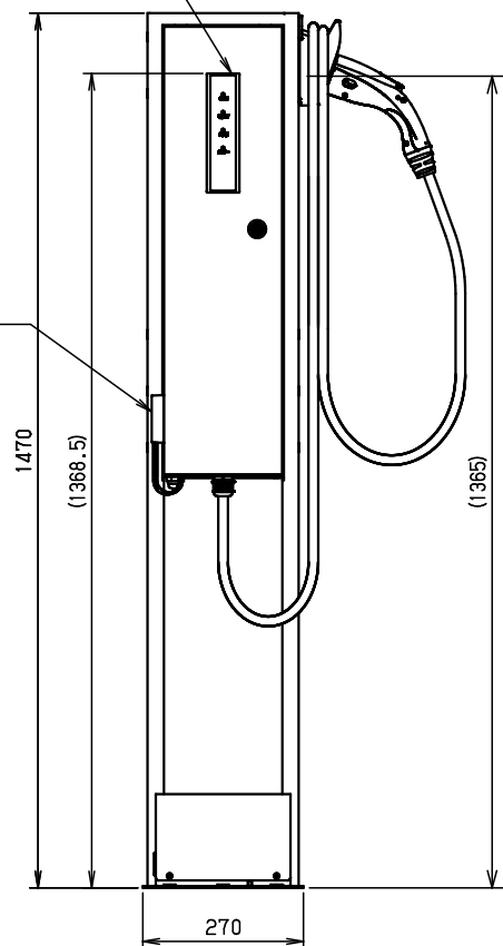
1台取付例
