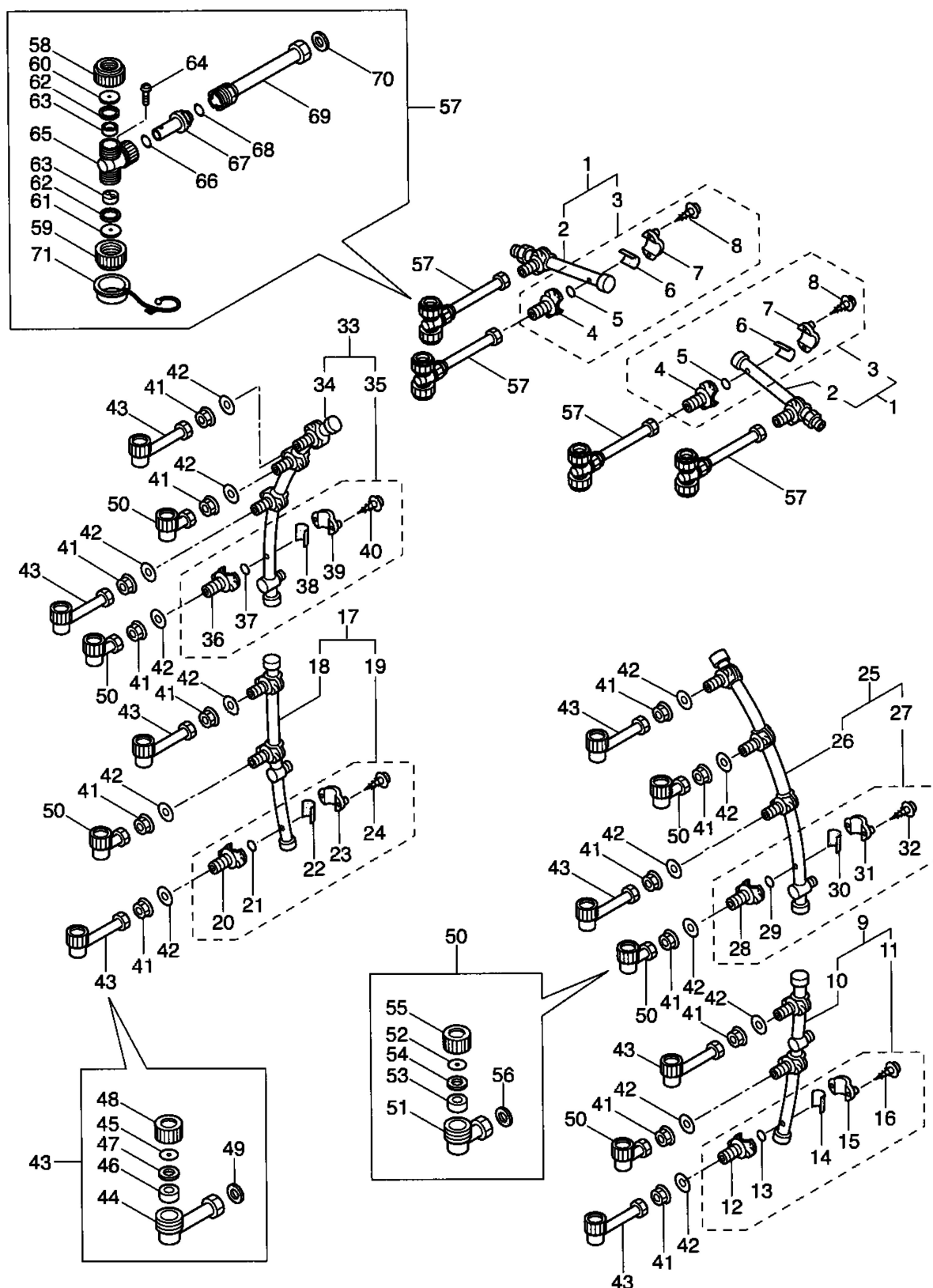
ノズル配列図
