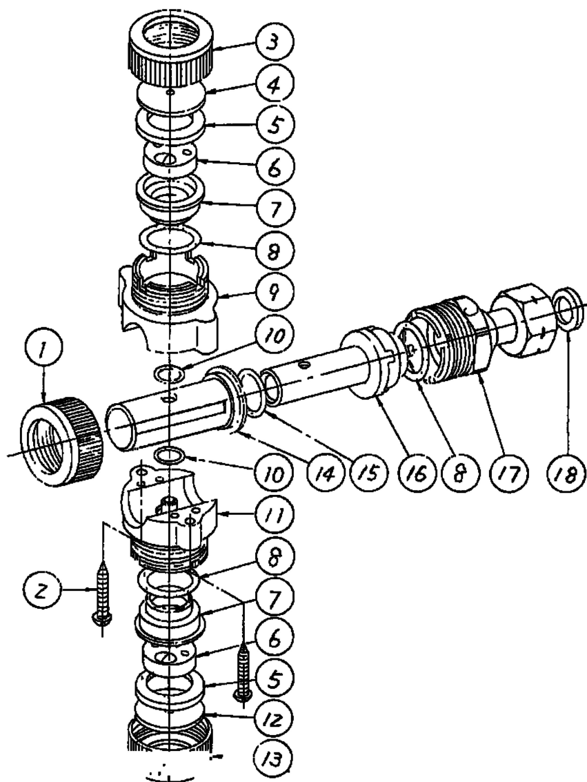
SSA-G530ノズル配列図 (SS用2方切替噴口)
