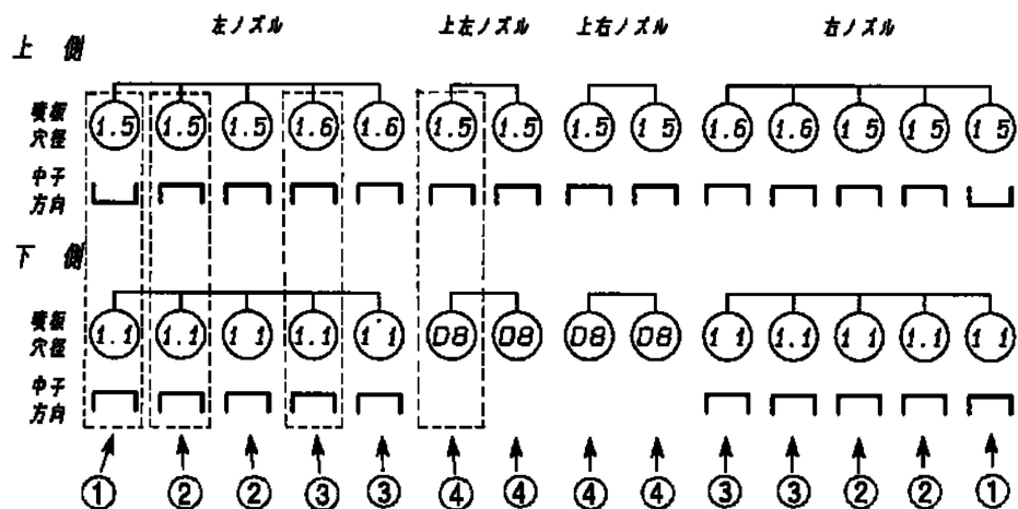
SSA-G530ノズル配列図 (SS用2方切替噴口)
