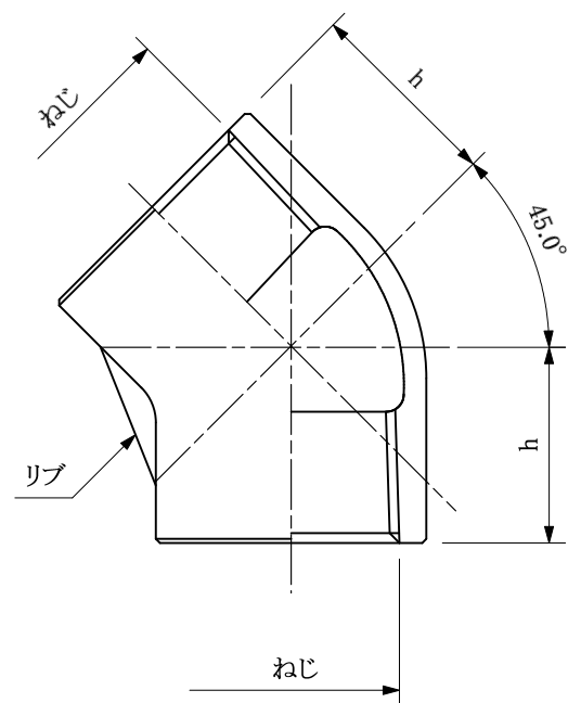
寸法表 (mm)
