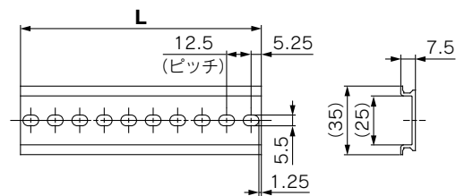
L寸法表 [mm]
