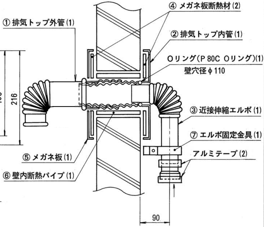
■ 設置図
