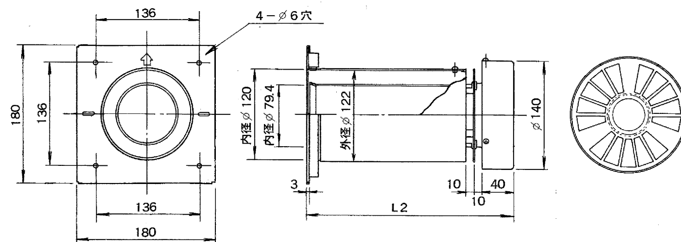
■給排気トップSET (SUS 304 t0.3~0.6)
