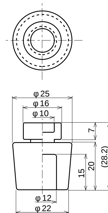
②BUAユニットバス用補助脚S（尺度1／1）
