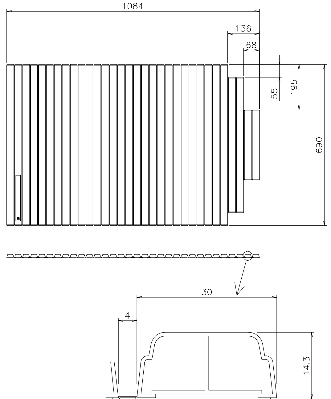
断面図
