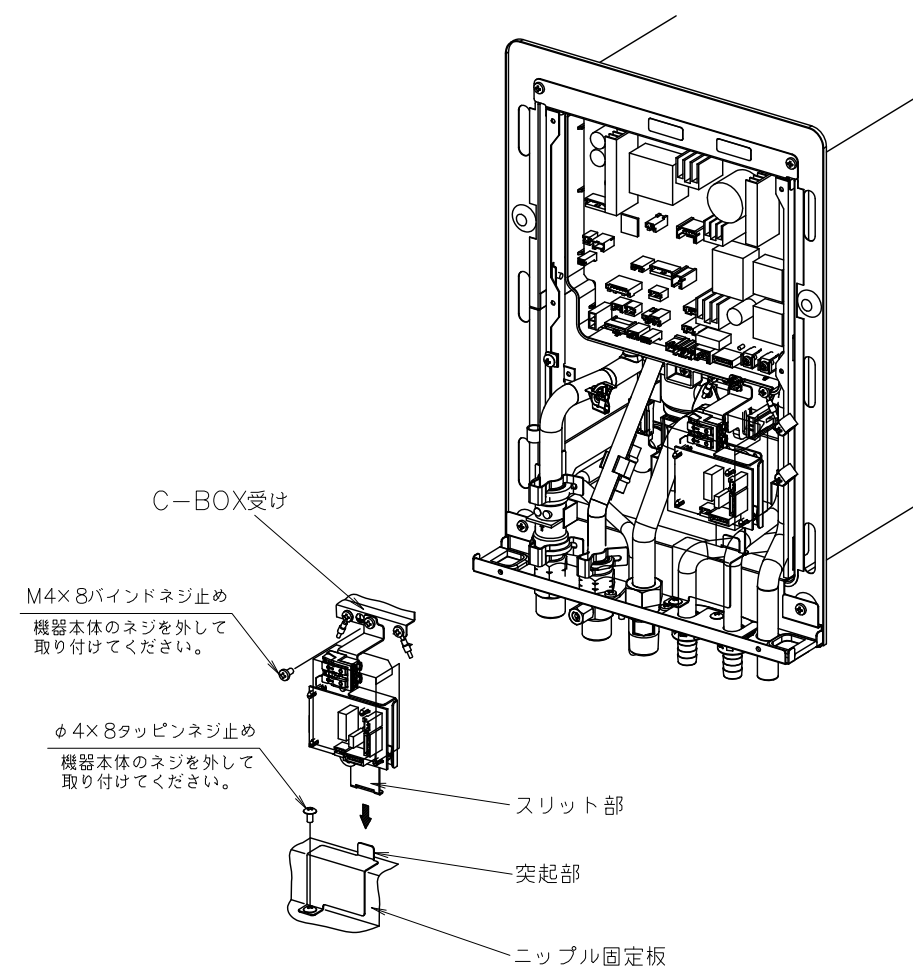
取り付け完成図（概略）
