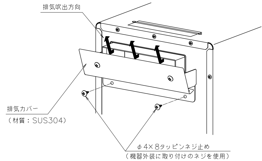
取り付け完成図 (概略)
