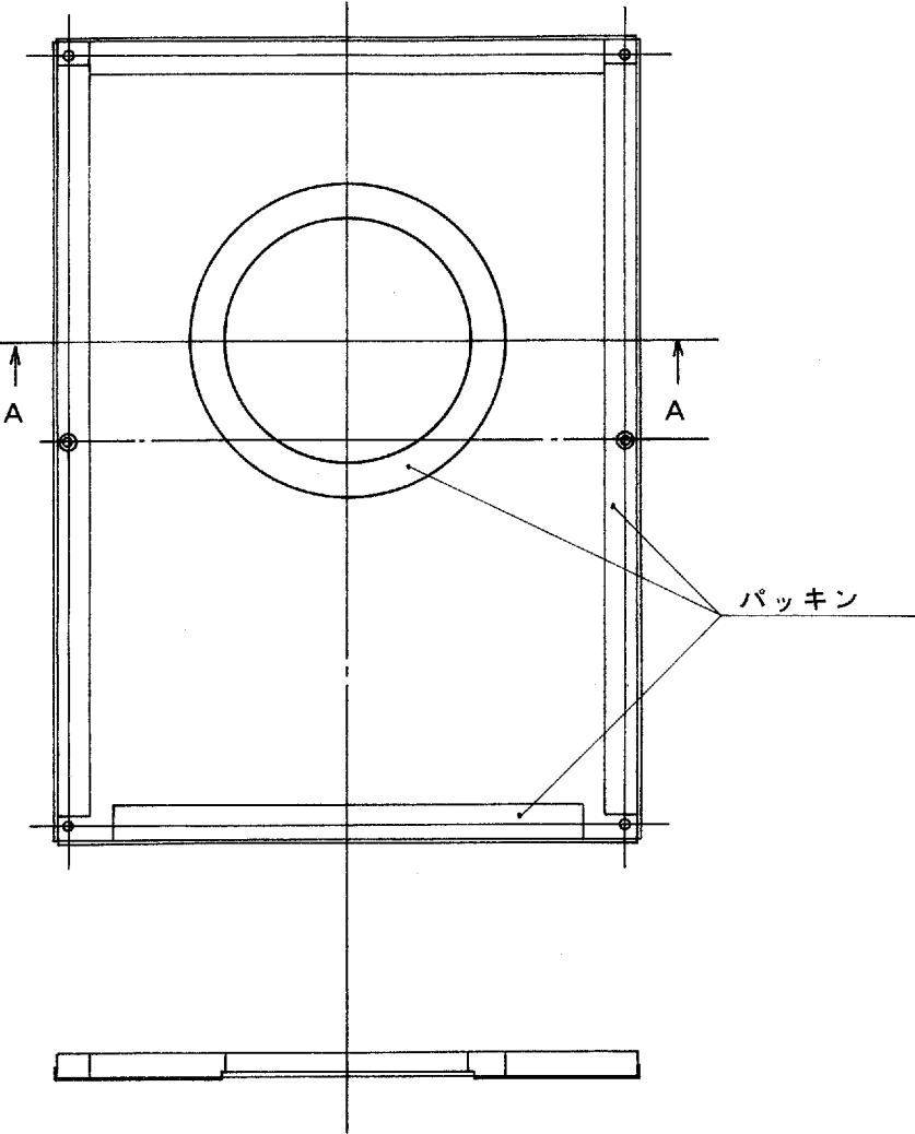
(断面 A-A')
